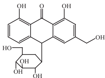
Aloin A
